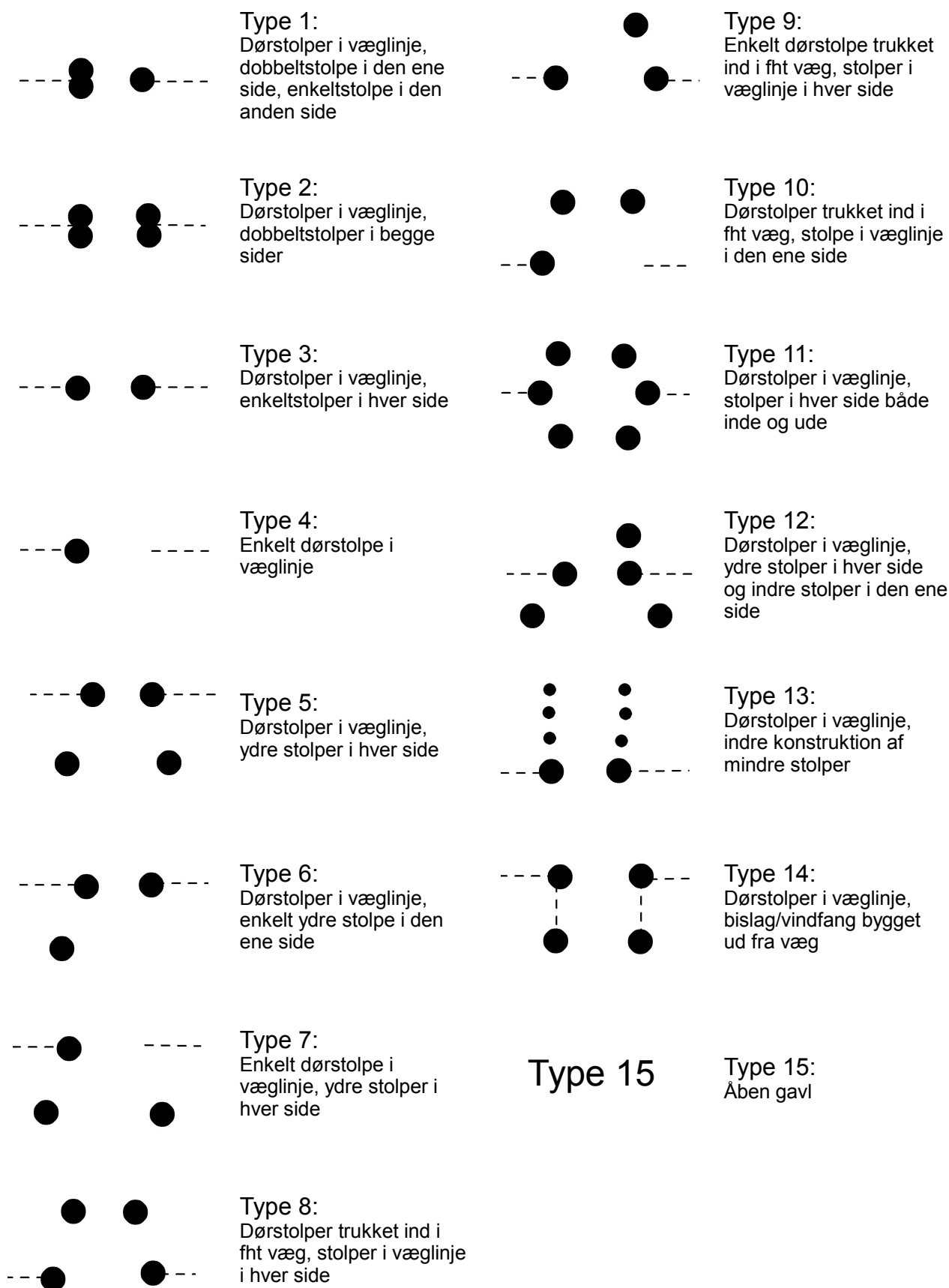
Fig. 13: Oversigt over forskellige typer af dørpartikonstruktioner Stiplet linje markerer hvor væglinjen er tolket
