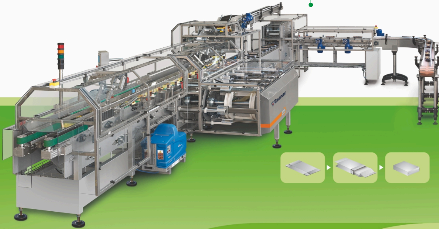
Encajadora horizontal de carga final continua, con amplio rango, de sistemas automáticos de alimentación. Soluciones de encajado económica y robusta, de alta flexibilidad.
