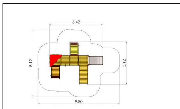
LM224 - Slide THEO
