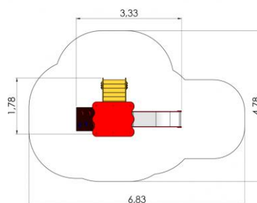
LM201PE - Slide EMMA
