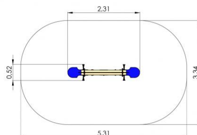
Nr. 10001 - Fjeder vippe
