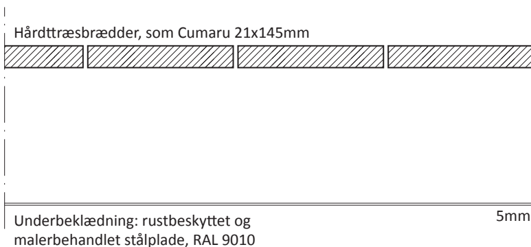
Lodret snit A-A 1:5
