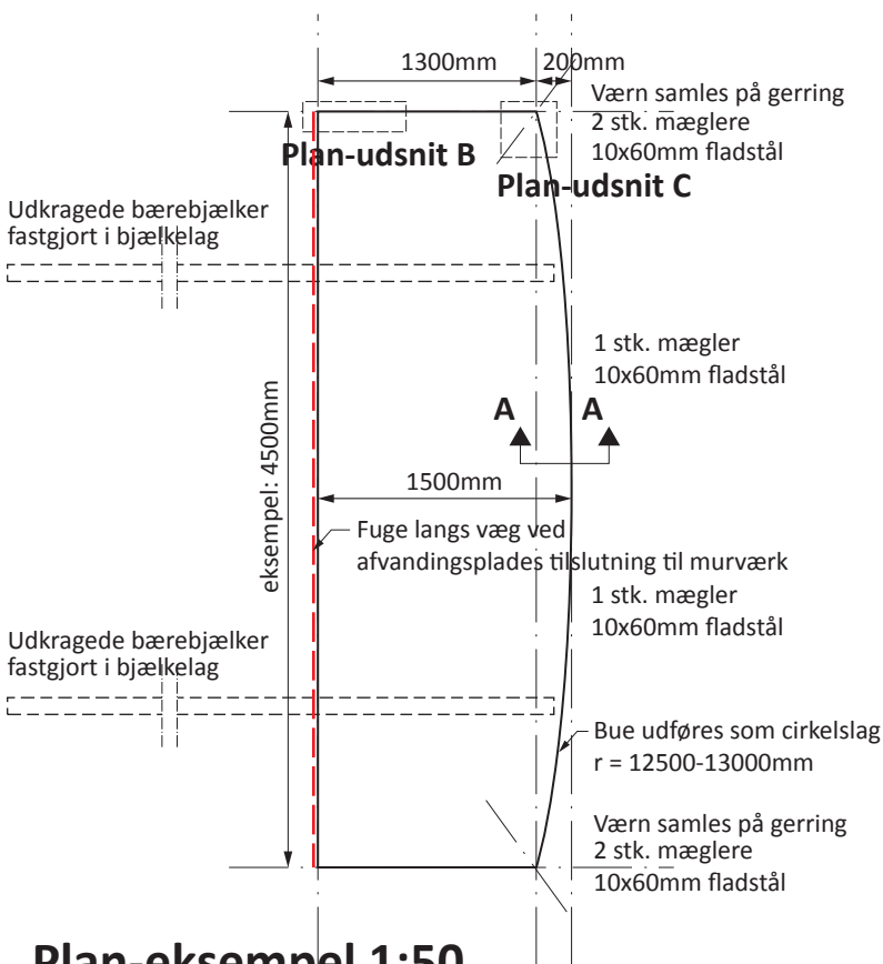
Plan-eksempel 1:50
