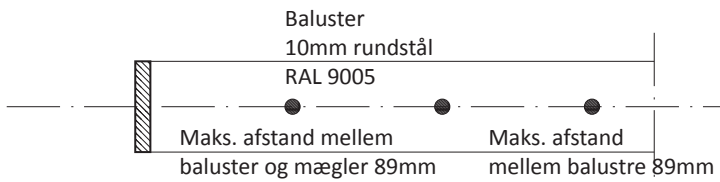
Plan-udsnit B 1:5
