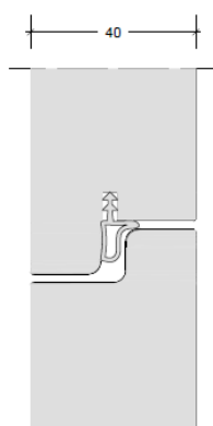
40 mm med tætning
