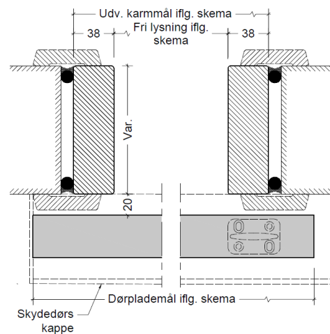
Blændkarm type 1 uden anslag
