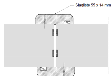
BD30/35dB + BD30/40dB + BD60/35 BD60/40dB dobbeltdør
