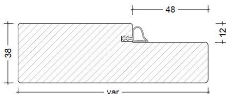
Standard karm med tætningsliste
