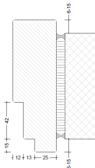
50mm karm med fremspring
