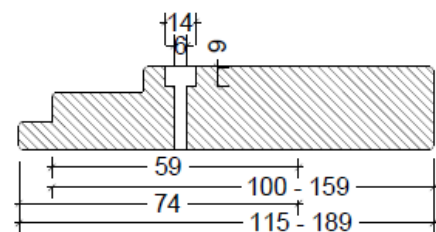
Illustration 3: Forboring af karm op til 159 mm
