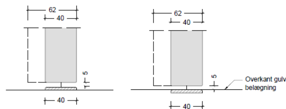
Rustfri stålskinne
