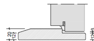
Træbund 62 mm dør
