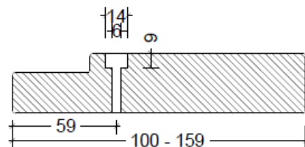
Illustration 1: Forboring af karm op til 159 mm
