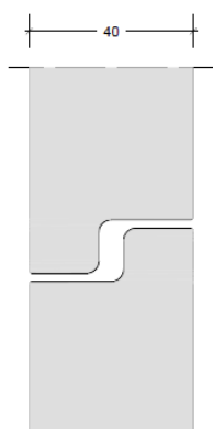
40 mm uden tætning
