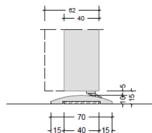
Gummibund og slæbeliste
