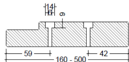
Illustration 2: Forboring af karm fra 160 mm
