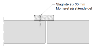
Uklassificeret dobbeltdør
