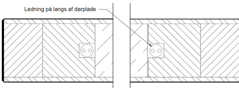
Vandret snit
