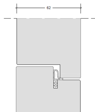
62 mm med tætning
