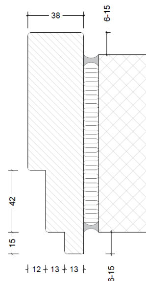
Karm med fremspring
