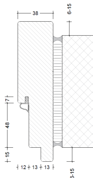
Karm med fremspring og tætningsliste
