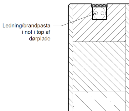
Lodret snit
