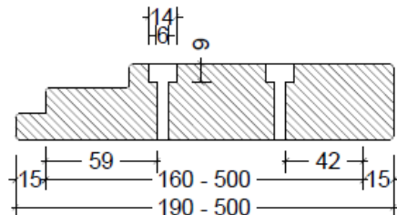
Illustration 4: Forboring af karm fra 160 mm
