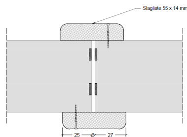
BD60 dobbeltdør
