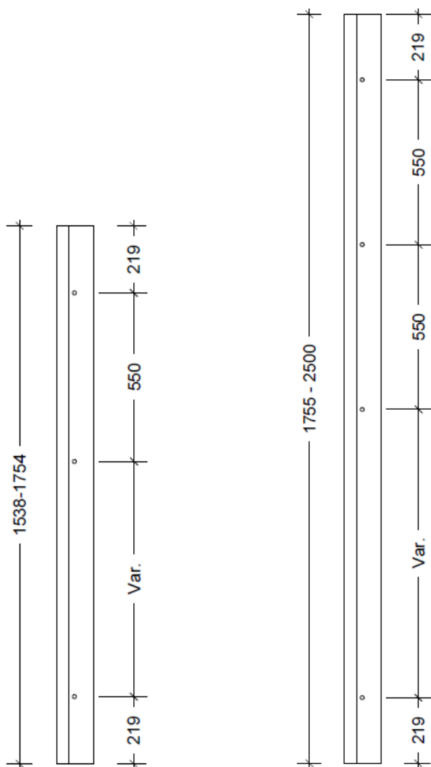
Placering af forboringer Udvendig karmhøjde 1538-1754 mm
