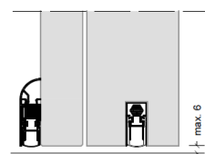
Bundløsning ved 49,7dB dør
