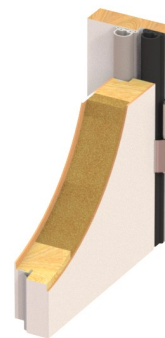
Snit af BD30/35dB klemfri dør
