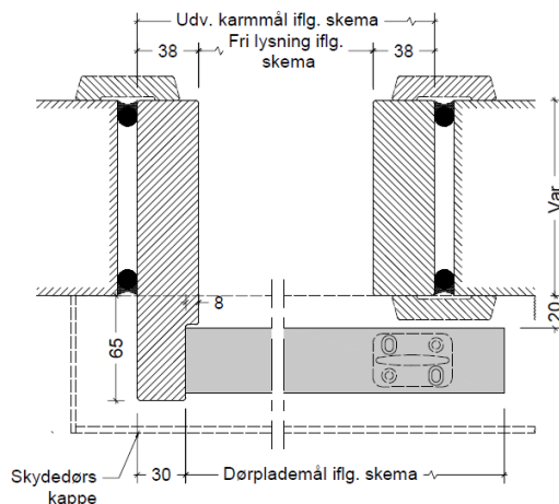
Blændkarm type 3 med anslag
