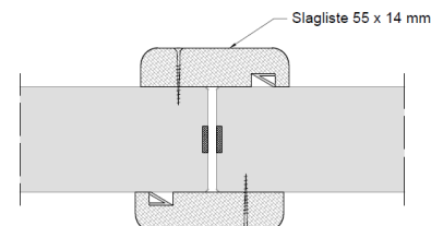
BD30/30dB + BD30/35dB dobbeltdør
