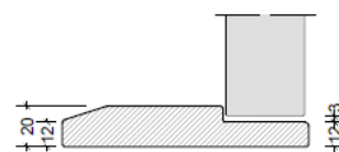
Træbund 40 mm dør
